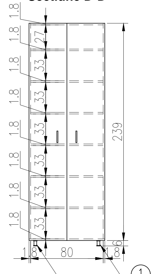
Sectione D-D
