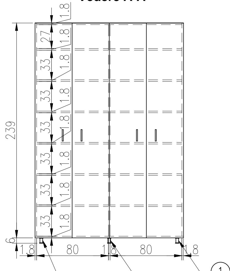
Vedere A-A
