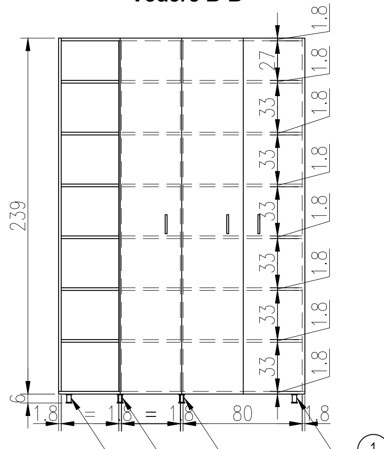
Vedere B-B
