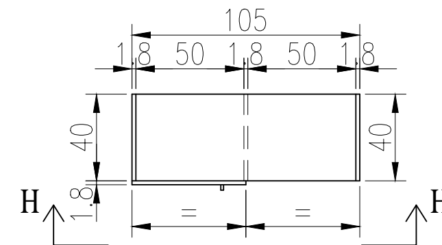
Vedere H-H
