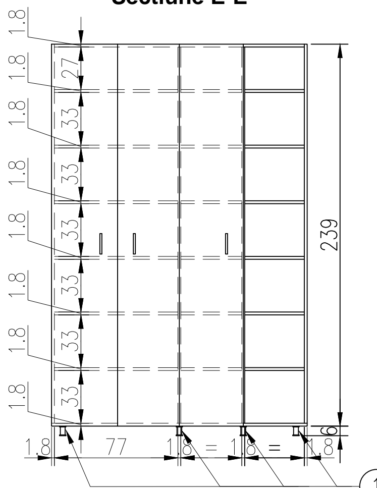
Sectione E-E
