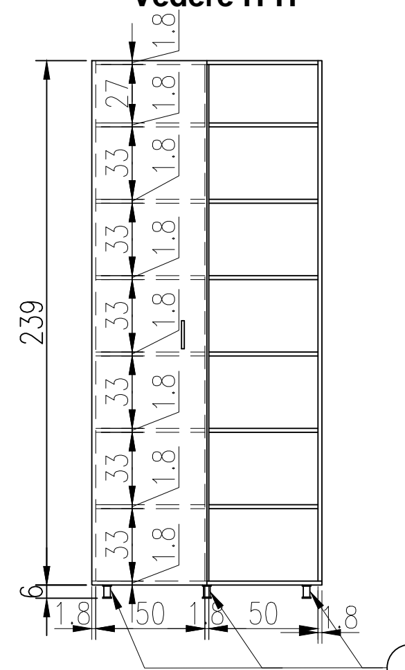
Vedere H-H
