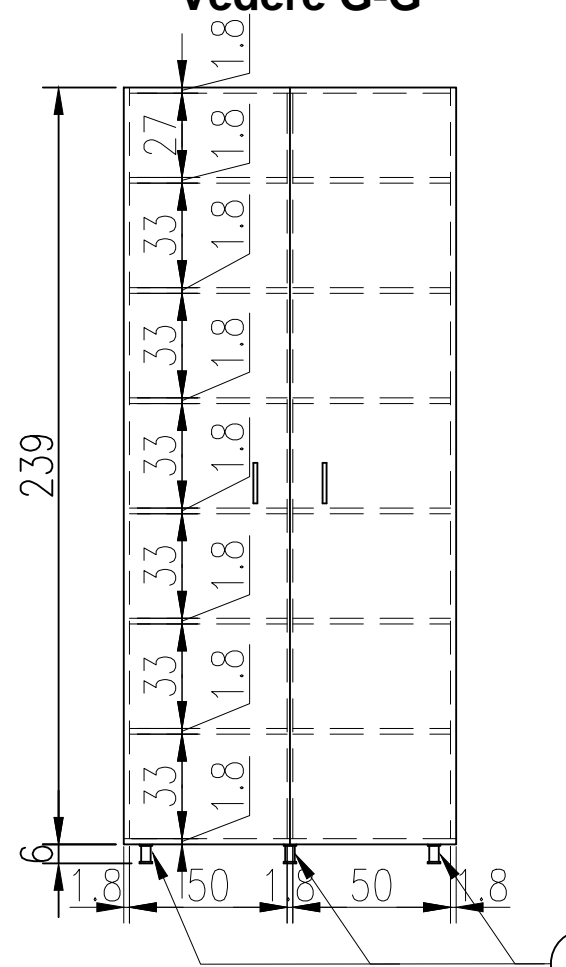
Vedere G-G
