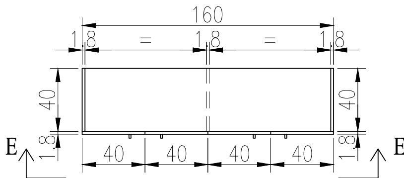
Sectione E-E
