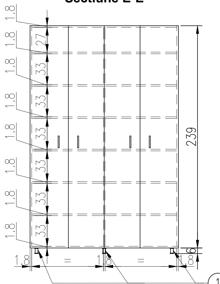
Sectione E-E
