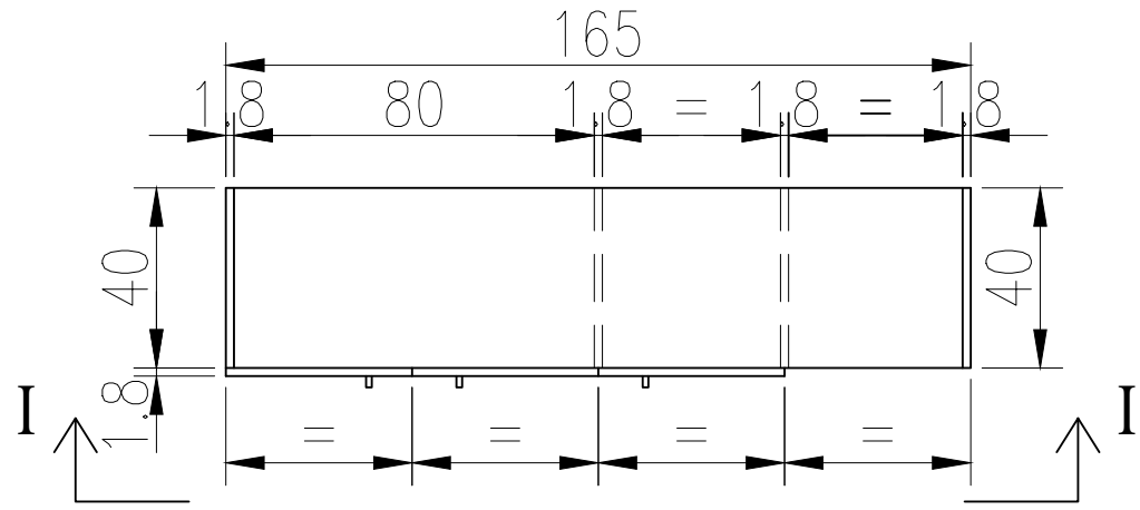
Vedere I-I
