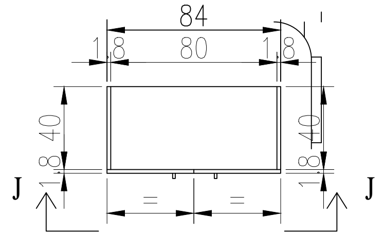
Sectione J-J
