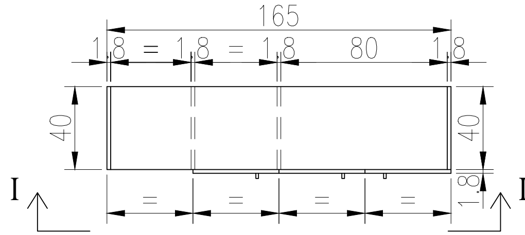
Vedere I-I
