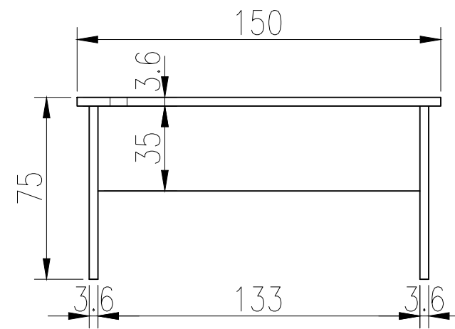
Vedere C-C
