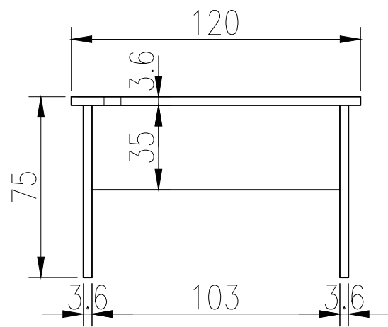
Vedere A-A
