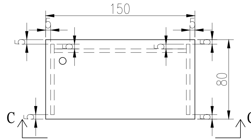
Vedere C-C
